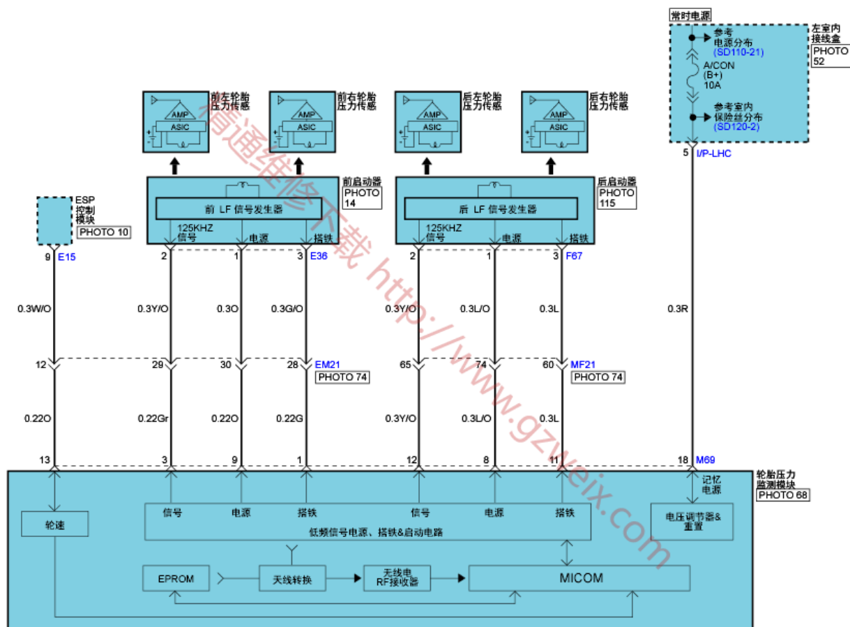
轮胎压力监测系统(TPMS) (2)
